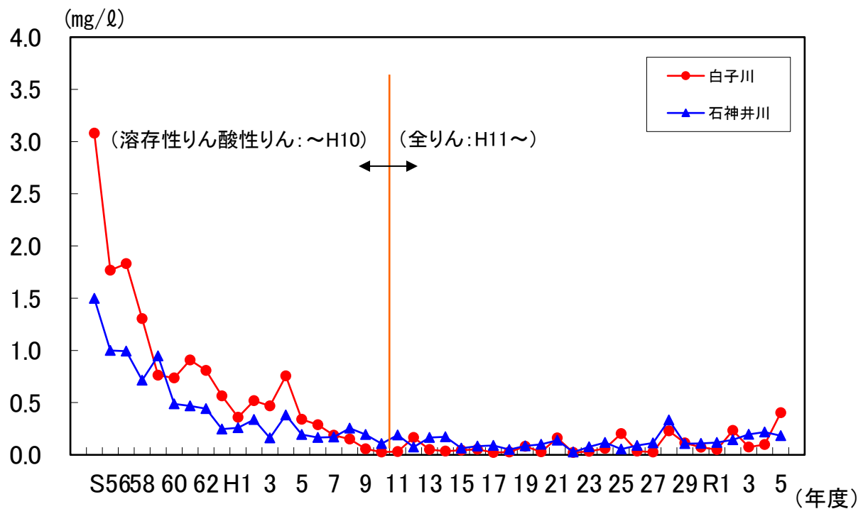
図17 白子川・石神井川の全りん(T-P)・溶存性りん酸性りん経年変化
