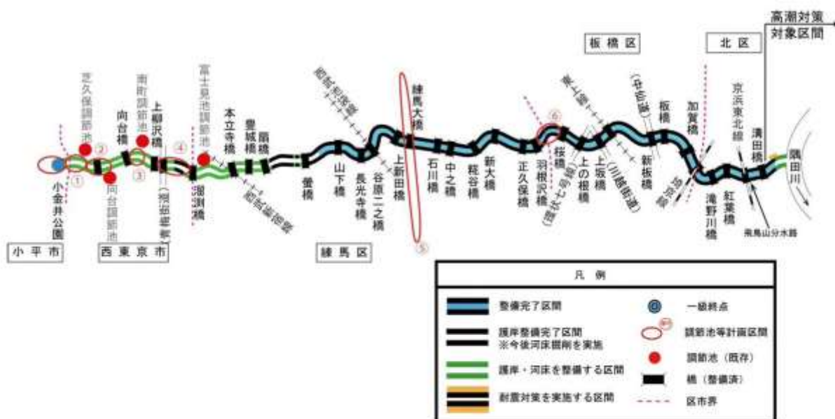
図 4-1 石神井川河川整備箇所図
