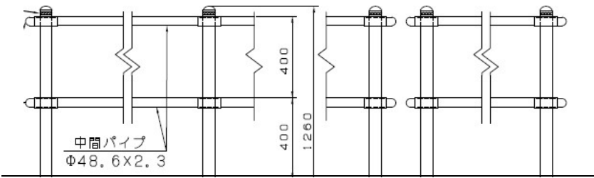
防護柵・横断抑止柵
