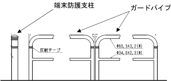
ガードパイプ・端末防護支柱
