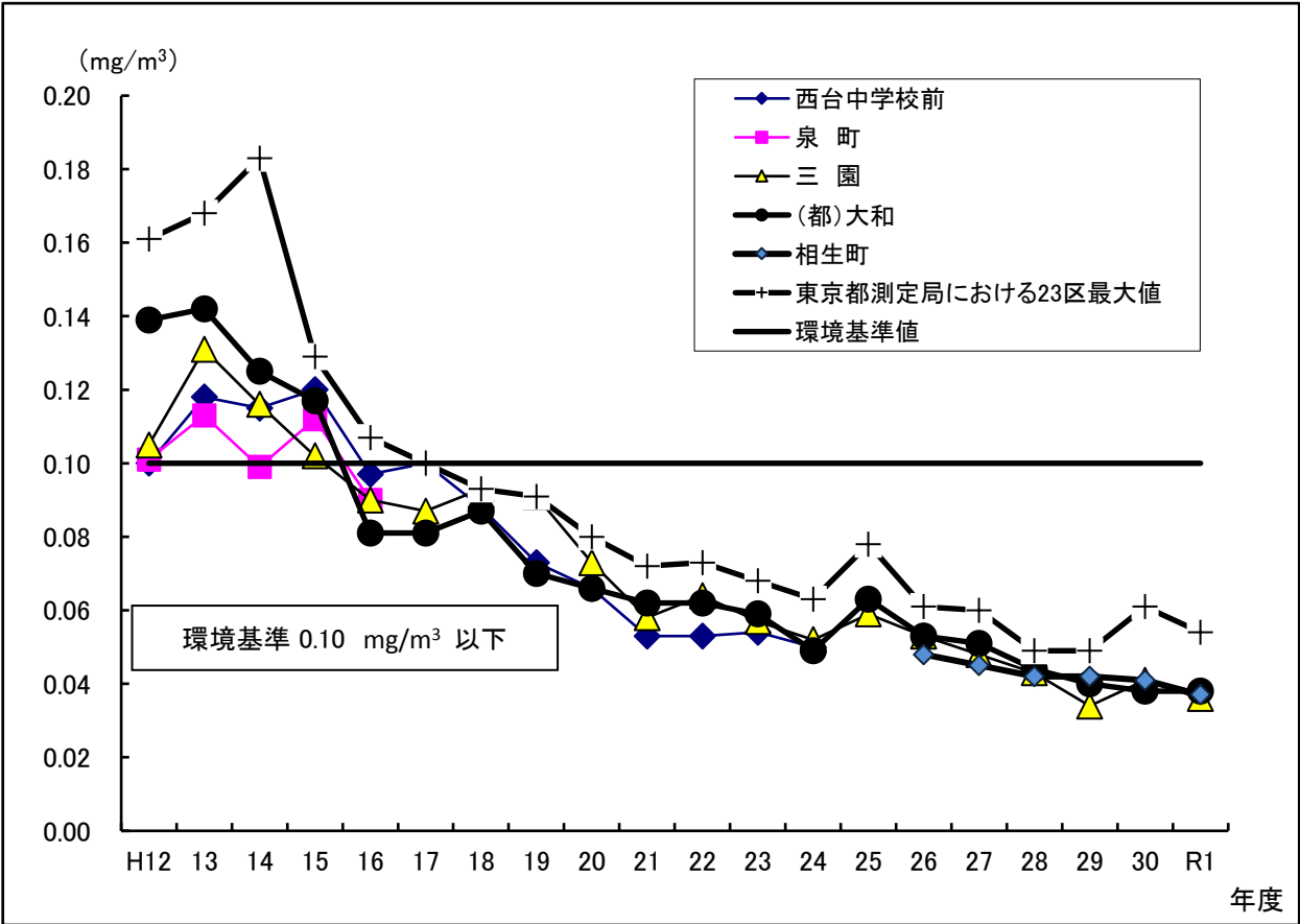
日平均値の2%除外値 (道路沿道測定室) の経年変化グラフ
