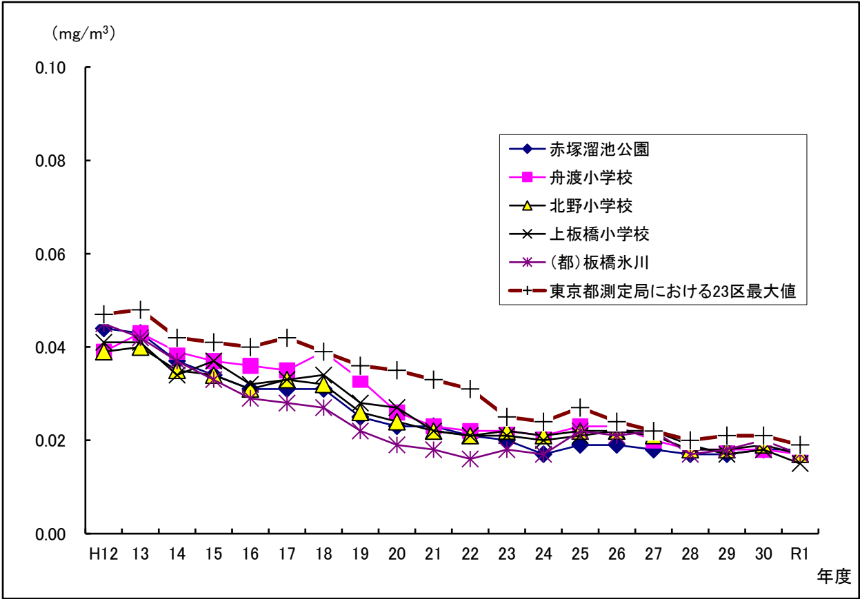
1時間値の年平均値（一般環境測定室）の経年変化グラフ
