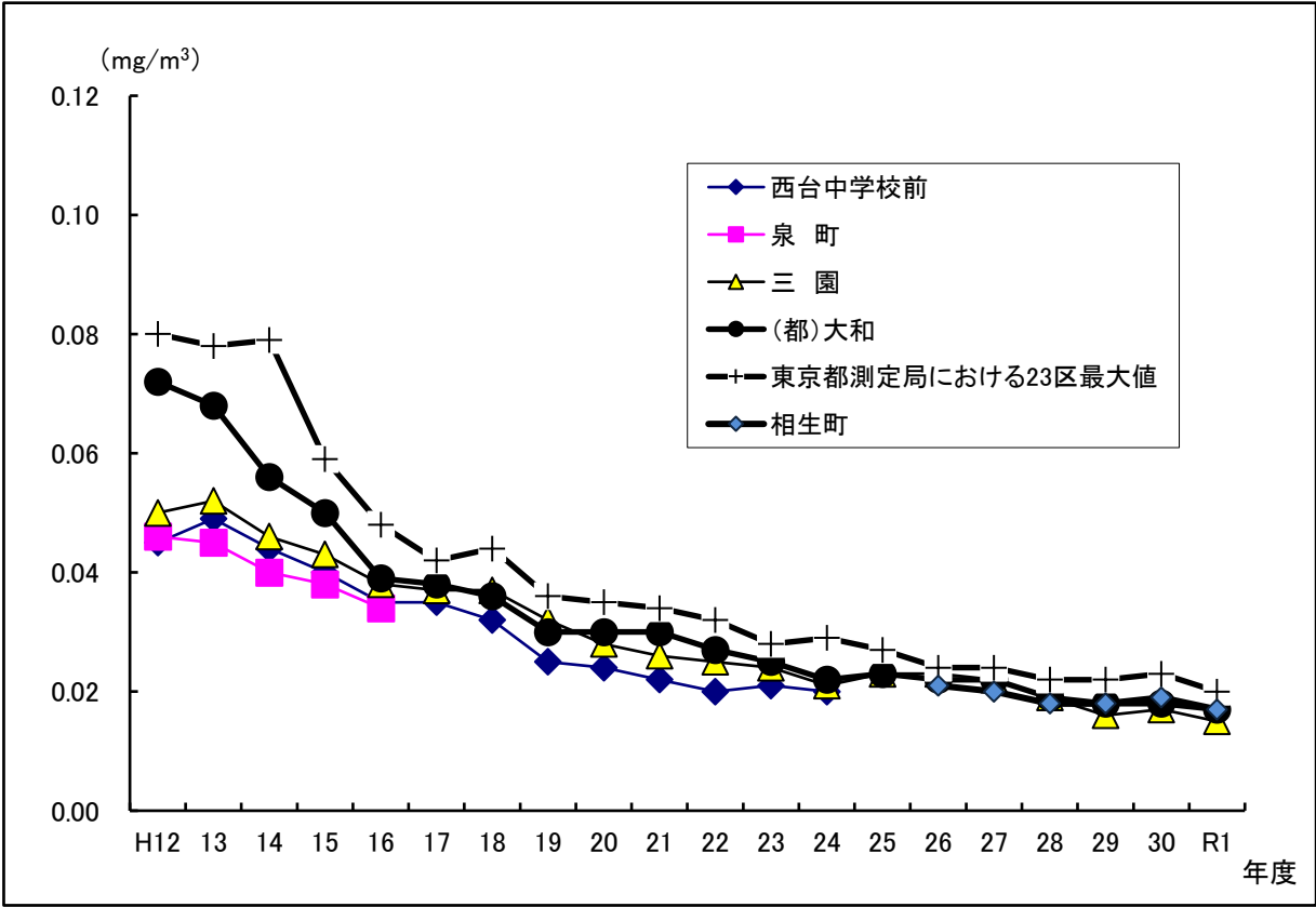
1時間値の年平均値(道路沿道測定室)の経年変化グラフ
