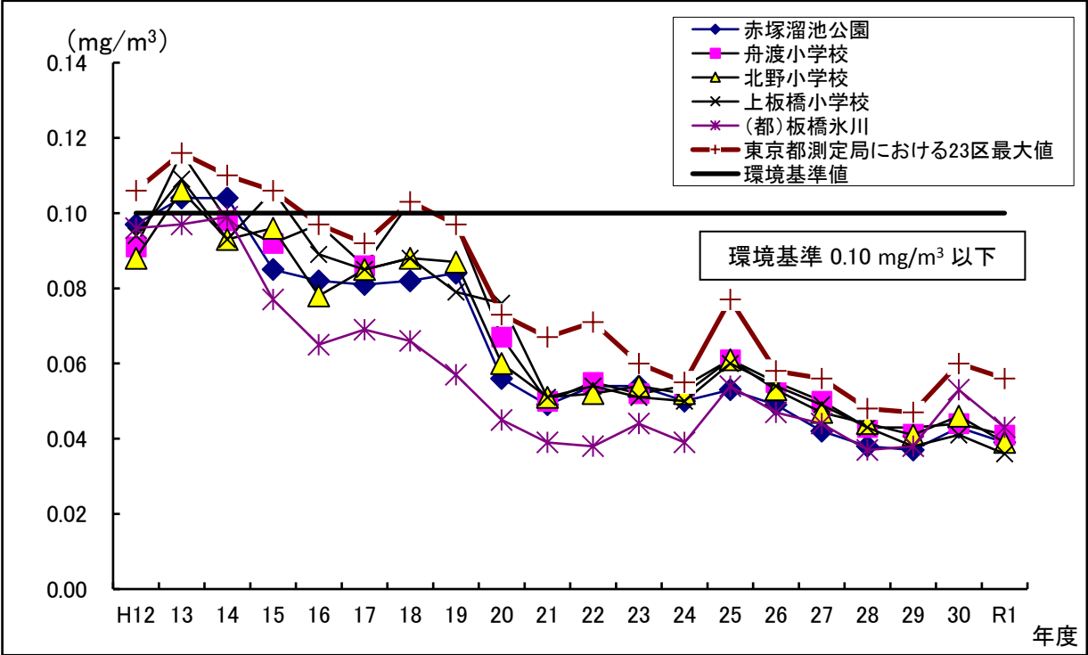
日平均値の2%除外値 (一般環境測定室) の経年変化グラフ
