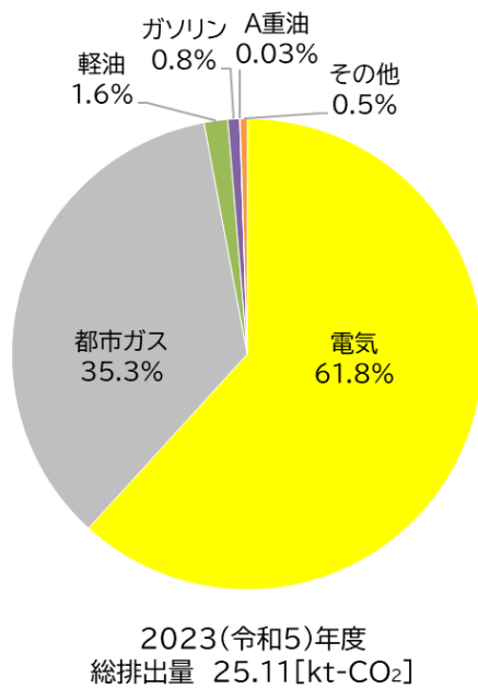
図1 エネルギー別の排出割合
