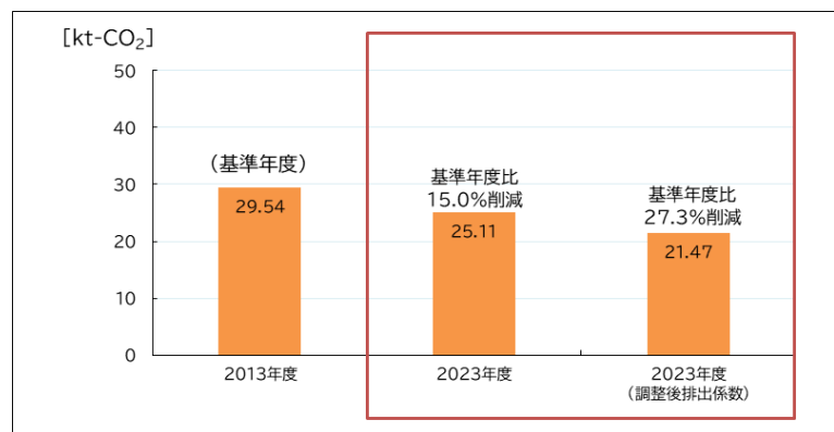
図2 温室効果ガス総排出量
