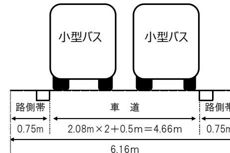
歩道がない単断面道路の例
